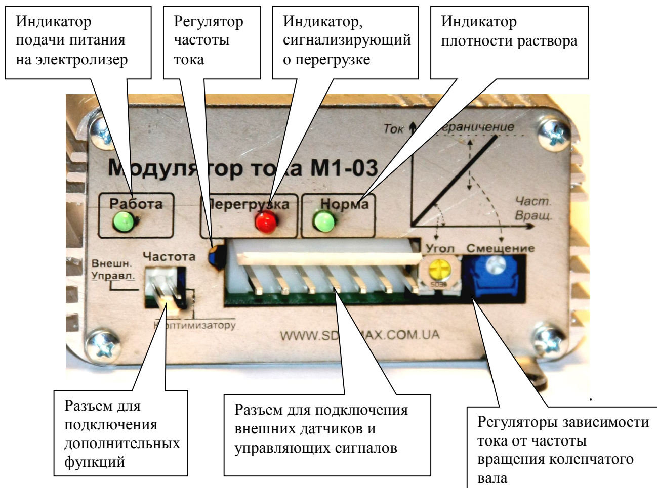
Рис.3.1. Внешний вид модулятора тока М1-03.
