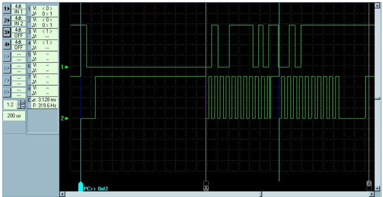
Рис. 2 Маркированная скриптом анализатора PS2 осциллограмма.
